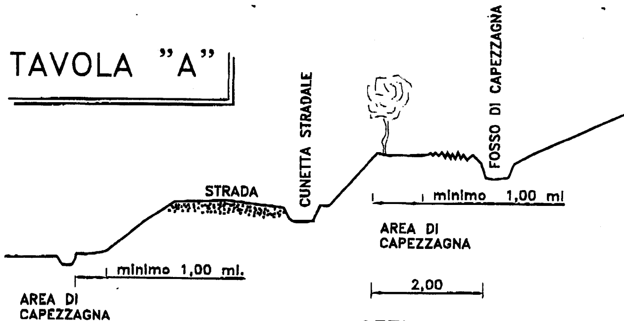
SEZIONE TRASVERSALE TIPO
